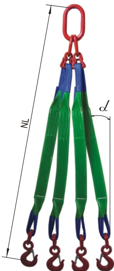
халка - куки
